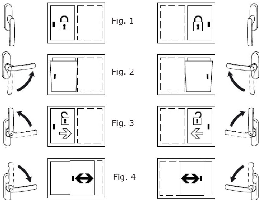
Fig. 1: Lukket position
