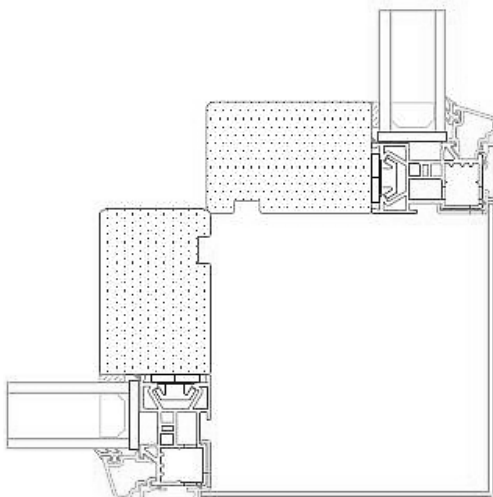
90° HJØRNELØSNING
