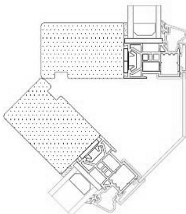
45° HJØRNELØSNING
